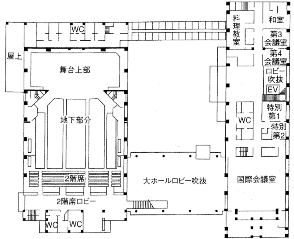
2階平面図
