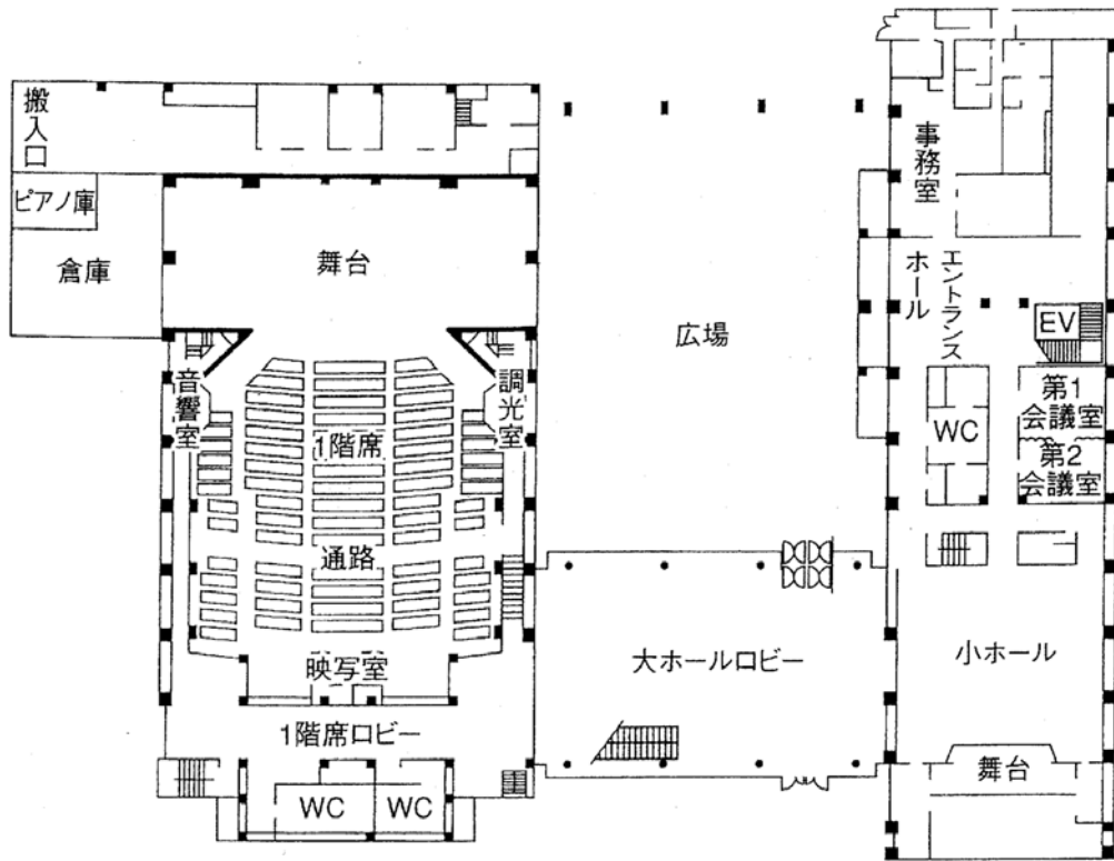
1階平面図
